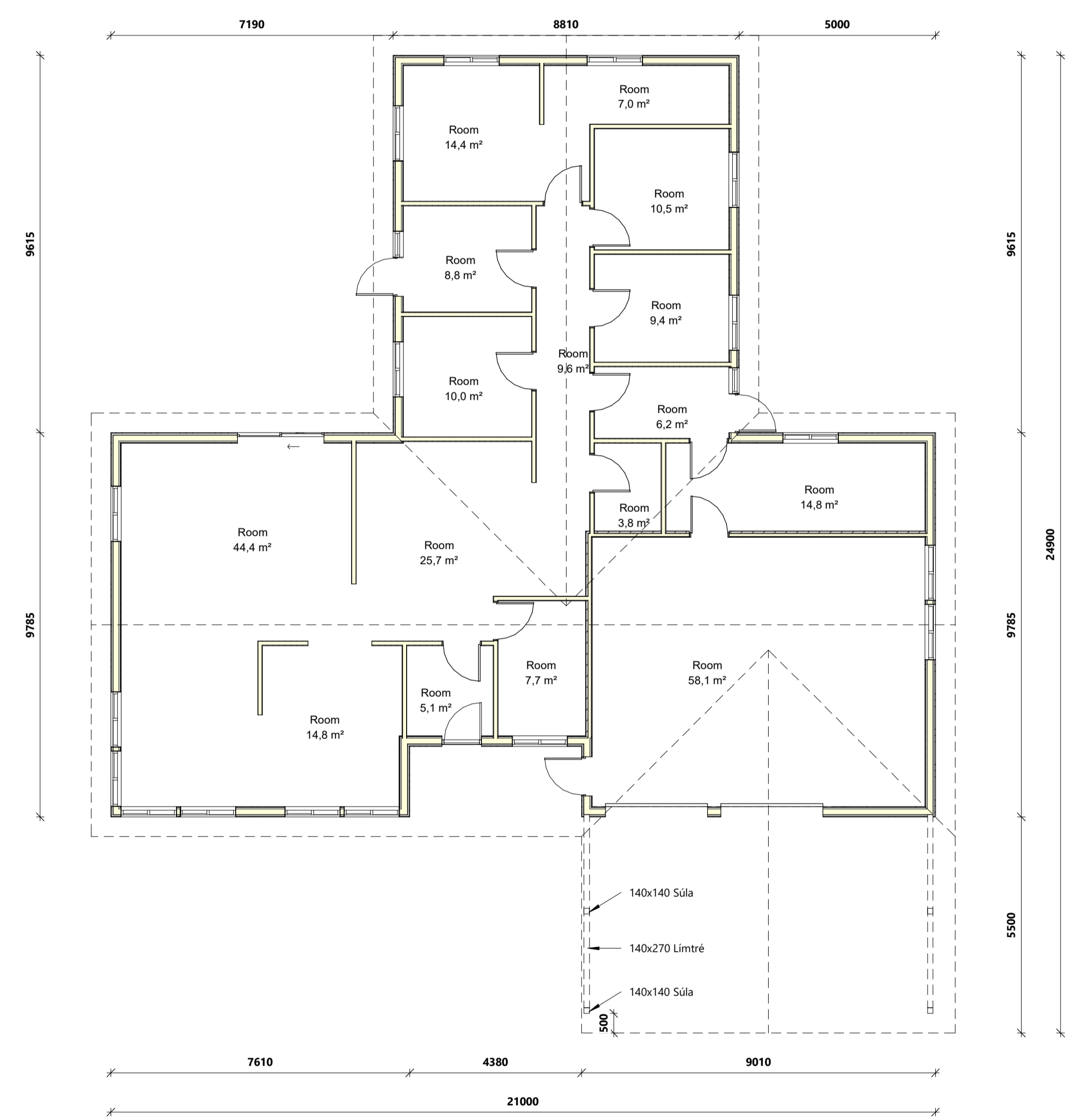
1 A- 1 hæð Grunnmynd 1 : 100
